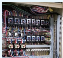
控制柜内设备异常发热
