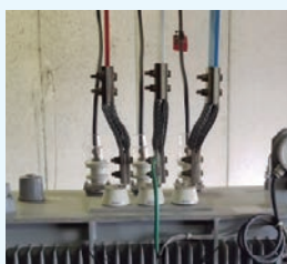
变压器异常发热
